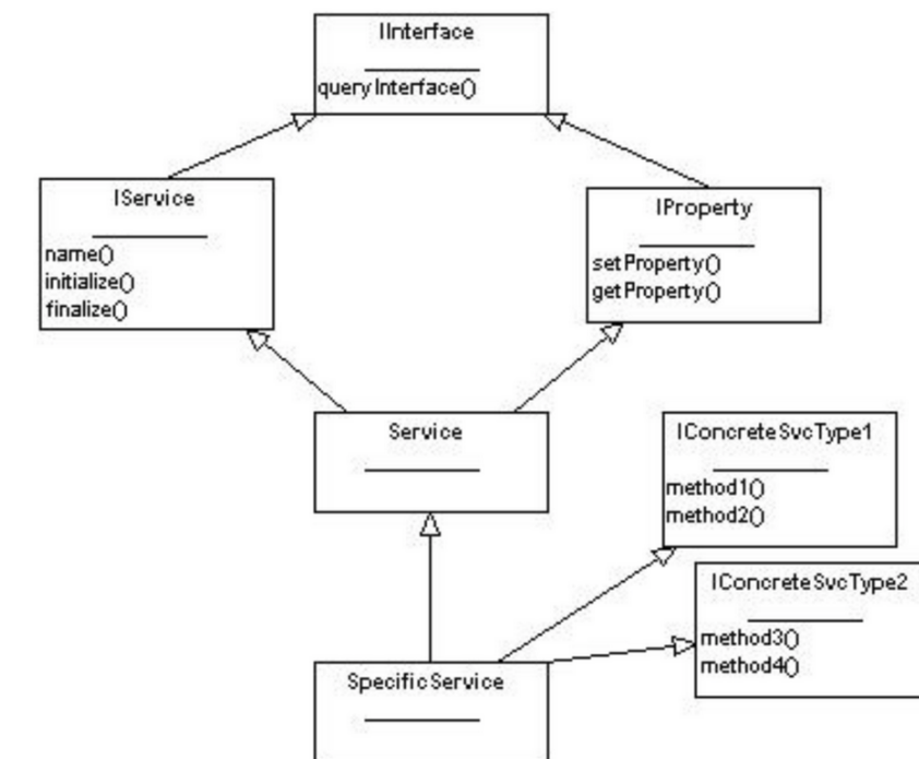
Рисунок 3.3 — Схема создания пользовательского сервиса.
