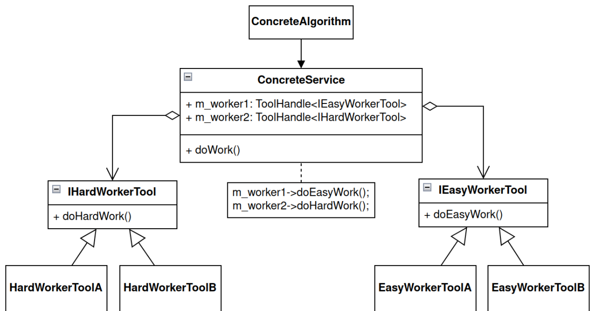
Рисунок 3.14 — Bridge в Gaudi
