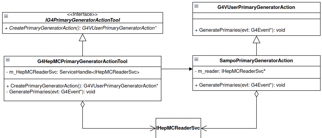
Рисунок 4.11 — Схема G4HepMCPrimaryGeneratorActionTool
