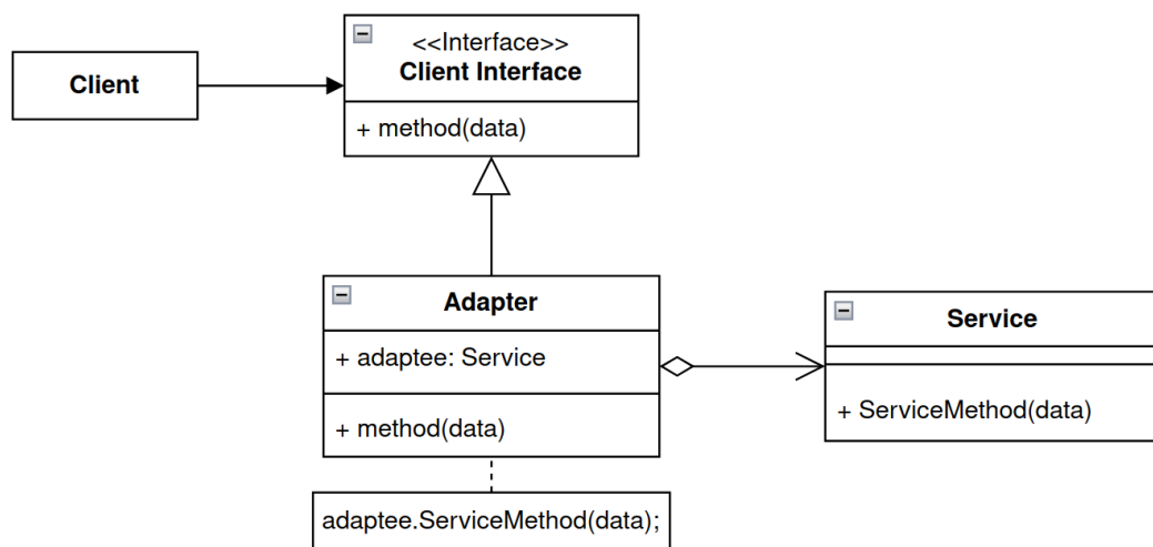
Рисунок 3.15 — Схема паттерна Adapter
