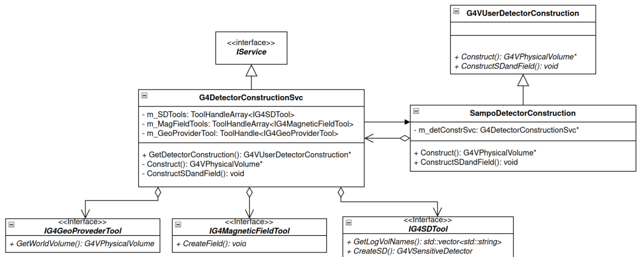
Рисунок 4.7 — Схема G4DetectorConstructionSvc
