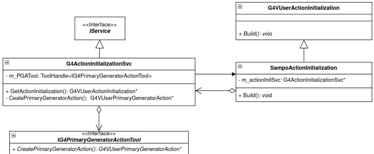
Рисунок 4.10 — Схема G4ActionInitializationSvc
