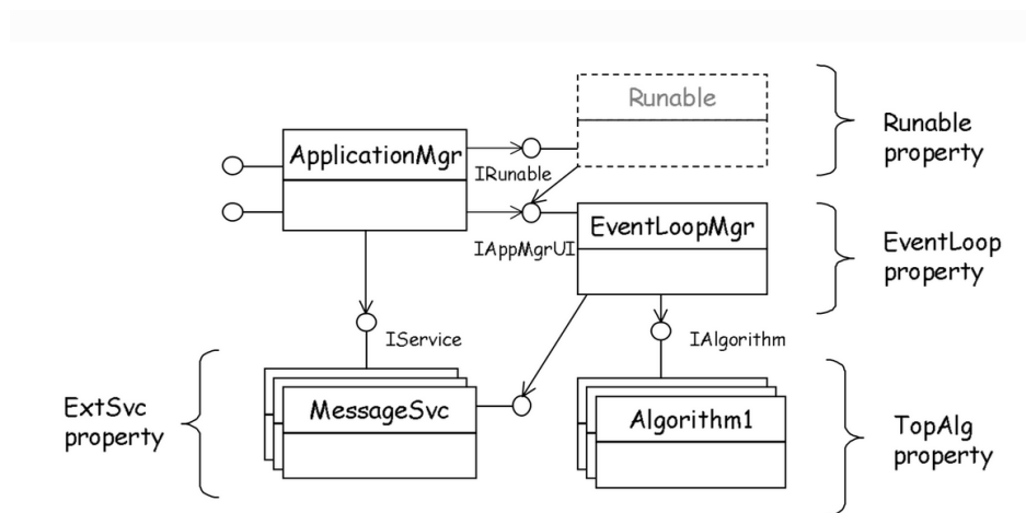
Рисунок 3.6 — Контроль и планирование в Gaudi.
